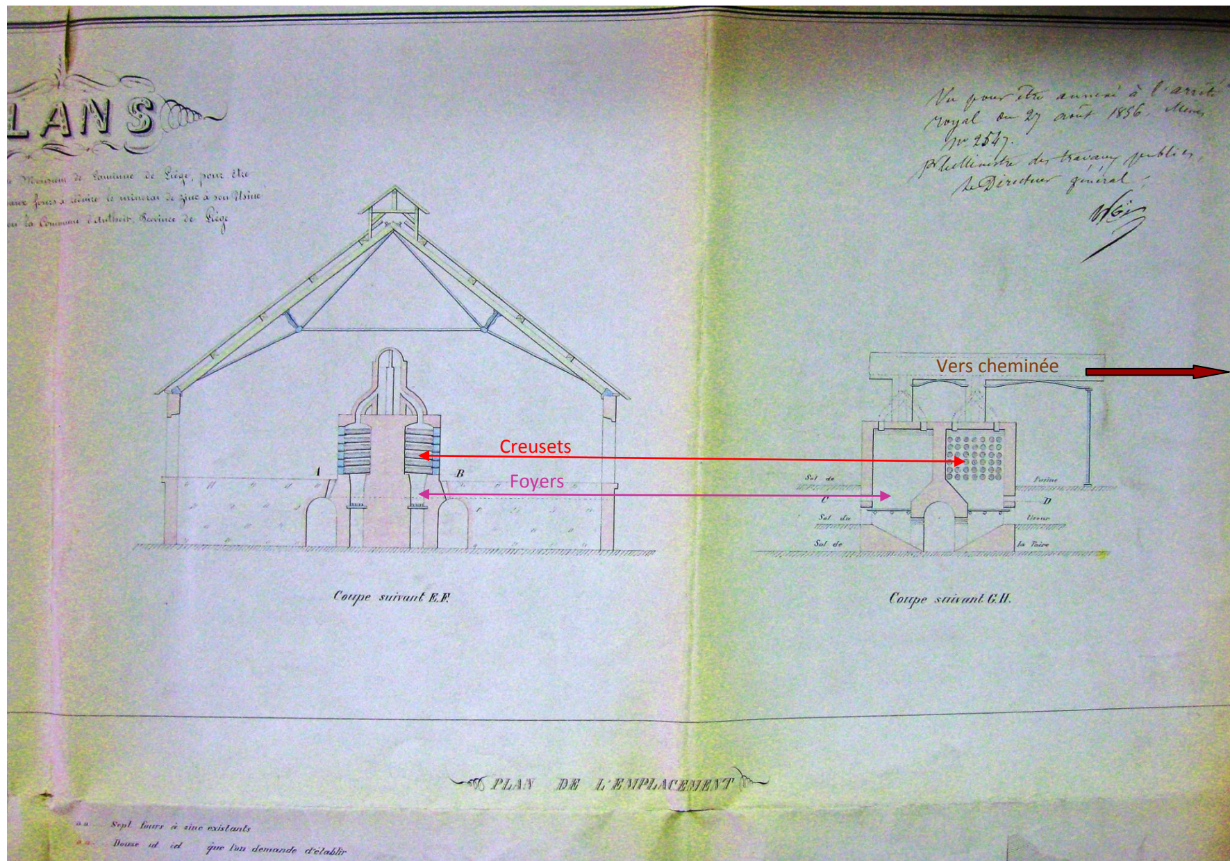
Extrait du plan de l'extension de l'usine à zinc
